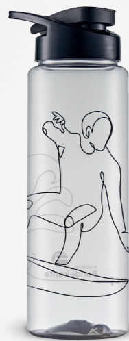
Cód. 1514 750 ml Diâmetro da Boca: 58 mm Diâmetro do Pote: 72,5 mm Altura do Pote: 235 mm EAN 13: 7896908215140 Caixa Master: 12 unid.
